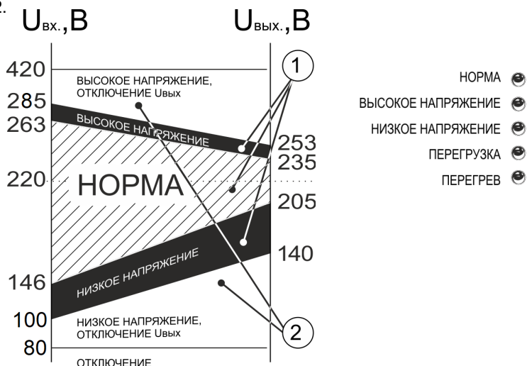
Рисунок 2 – Работа светодиодной индикации стабилизатора (1 – зона работающей нагрузки, светодиод «НОРМА» горит; 2 – зона отключения нагрузки, светодиод «НОРМА» мигает)
