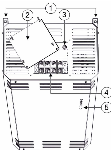
Рисунок 1. Общий вид стабилизатора и его функциональных элементов
