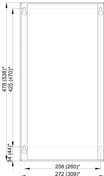
Рисунок 4 – Крепление прибора на стену, размеры со звездочкой* для исполнения ST-20000 , ST-30000
